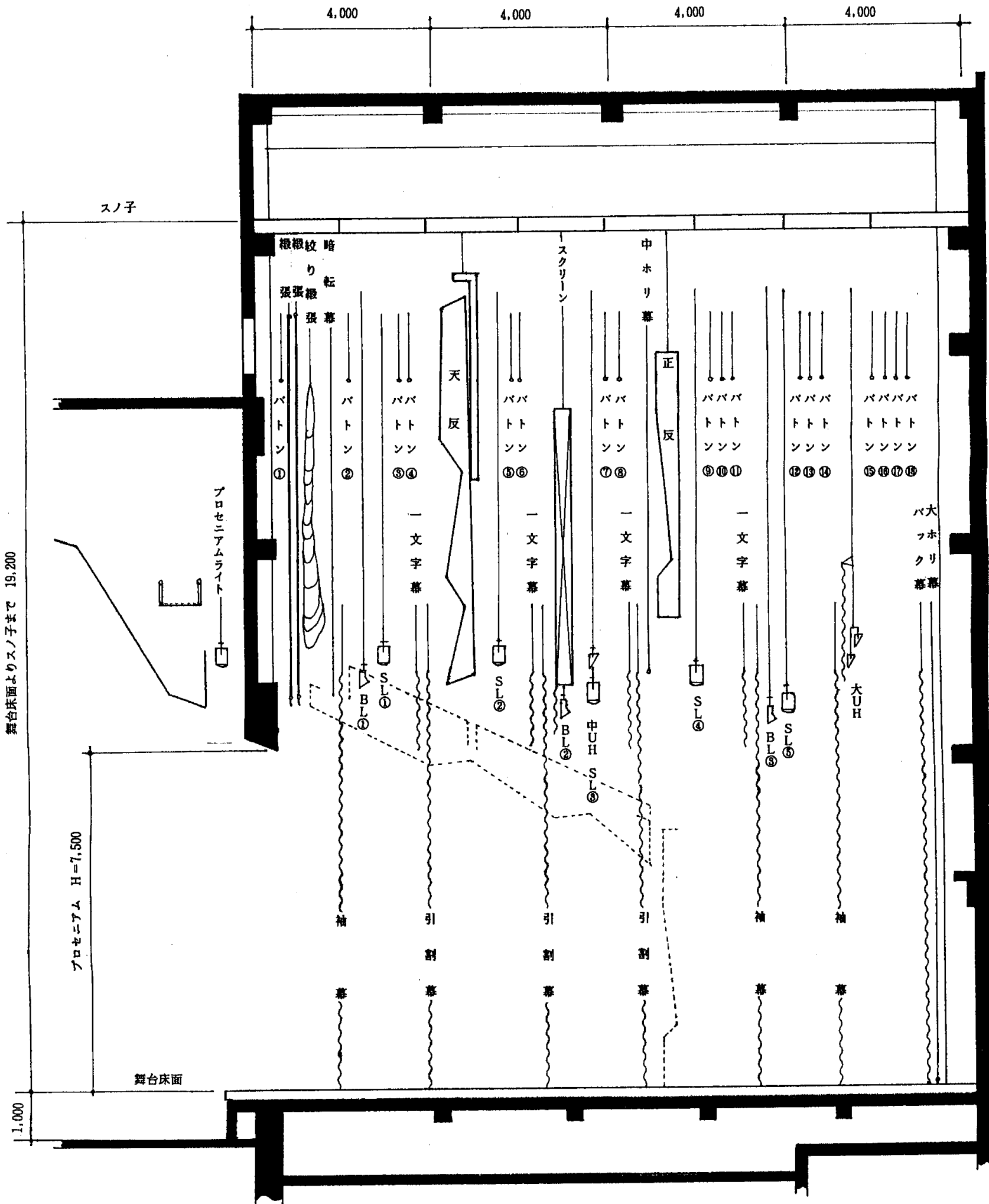
郡山市民文化センター 中ホール 舞台断面図
